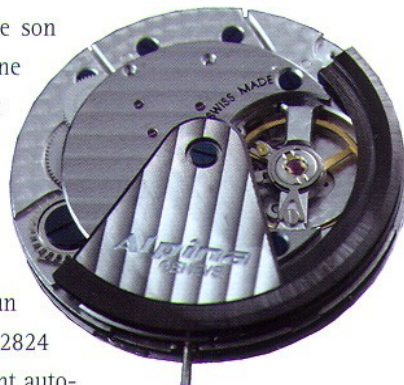
Ci-dessus: Le calibre automatique AL-700, spécifiquement développé «in house» pour la marque Alpina.
